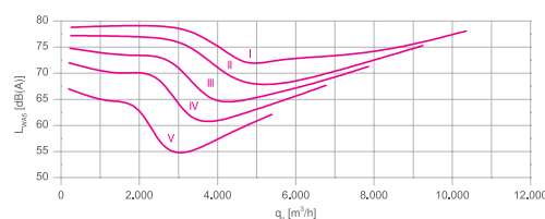
Charakteristika RH50V-4DK.6K.VR, 50Hz, 4-pólová
