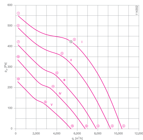
Charakteristika RH50V-4DK.6K.VR, 50Hz, 4-pólová
