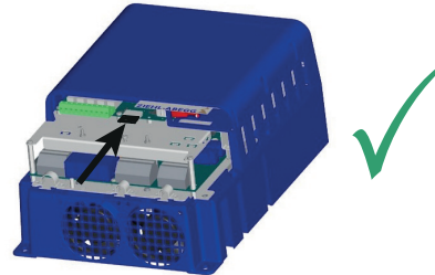
Speicherkarte im Kartenslot X-MMC bei ZAdyn4C 011-032
